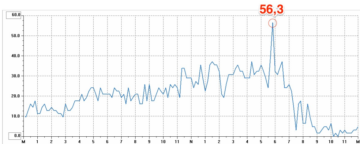
Ráfagas de viento registradas en ALCOSSEBRE entre el 11/11/22 (en km/h) https://inforatge.com/meteo-alcalaxivert
