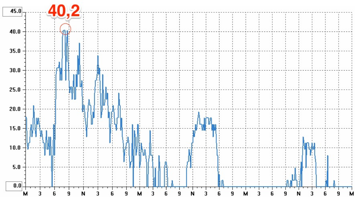
Ráfagas de viento registradas en ALCALÀ DE XIVERT entre el 12/11/22 (en km/h) https://inforatge.com/meteo-alcalaxivert
